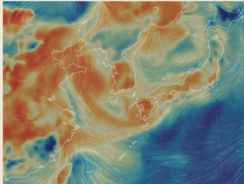
図1：3月末のPM2.5飛散状況(ECMWF)
